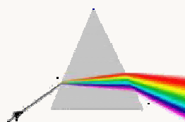
色散
